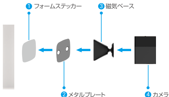
図1 フォームステッカーによる取り付け
