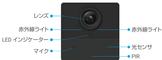
前面図
