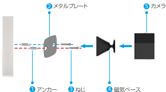
図2 ねじによる取り付け
