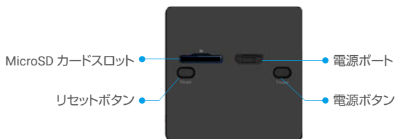
背面図
